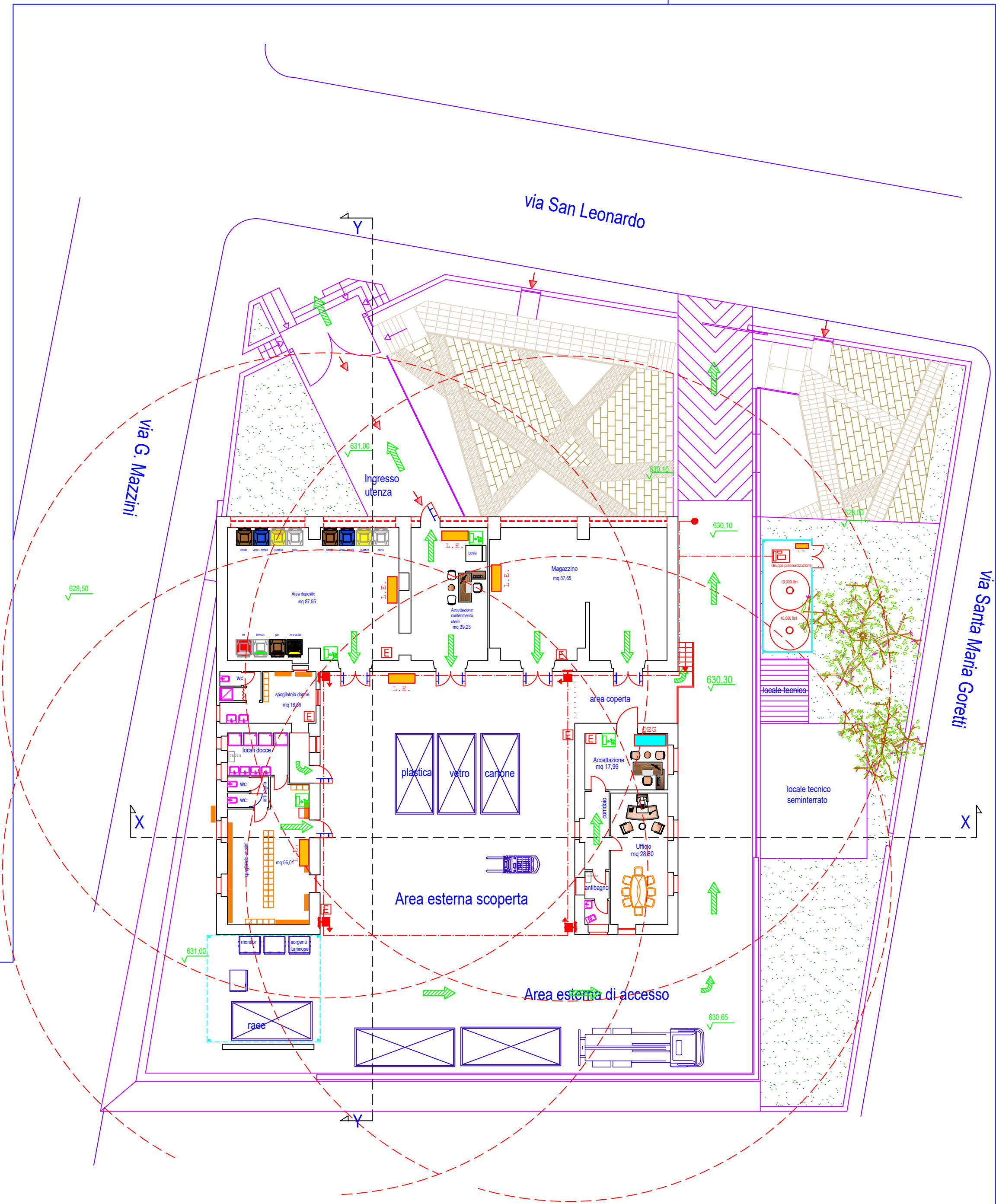
Planimetria impianto idrico e misure di sicurezza antincendio
